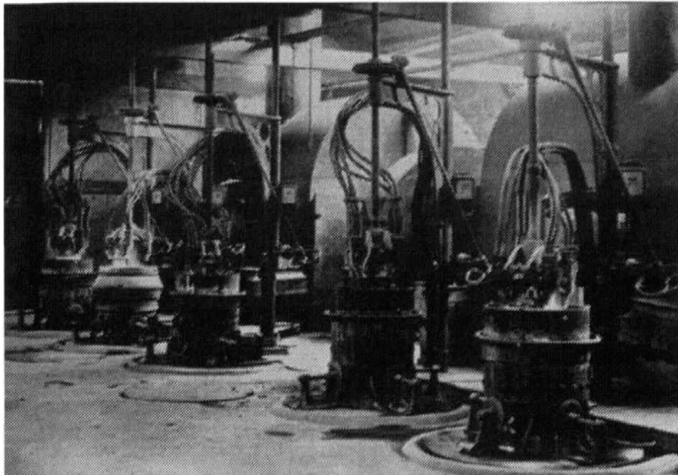
Produktionshalle der Société Electrométallurgique de Froges, um 1889 (© Institut pour l'Histoire de l'Aluminium)
