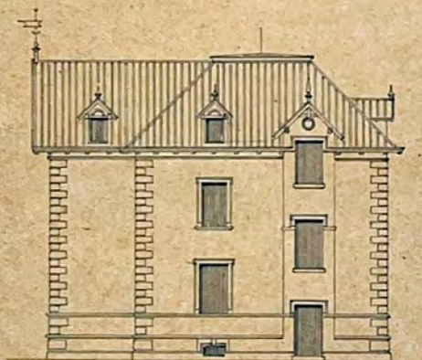
NORDFACADE
